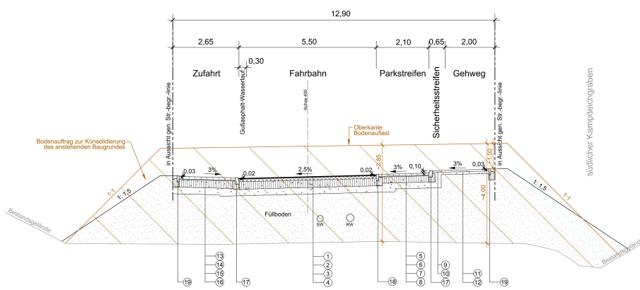
Schnitt B-B Planstraße C - Achse 400
