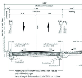
Ausbauquerschnitt II - II
