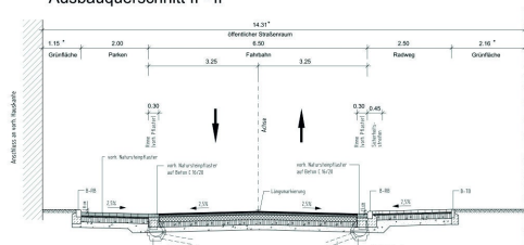
Ausbauquerschnitt II - II
